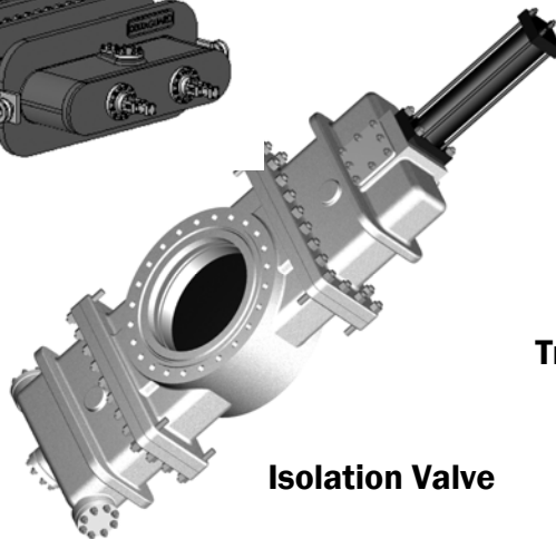
Bottom Unheading
